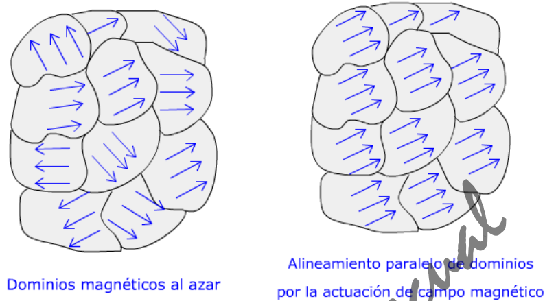
Figura 16.1.- Esquema mostrando los dominios magnéticos al azar (izquierda) y la alineación de los dominios magnéticos (derecha)
