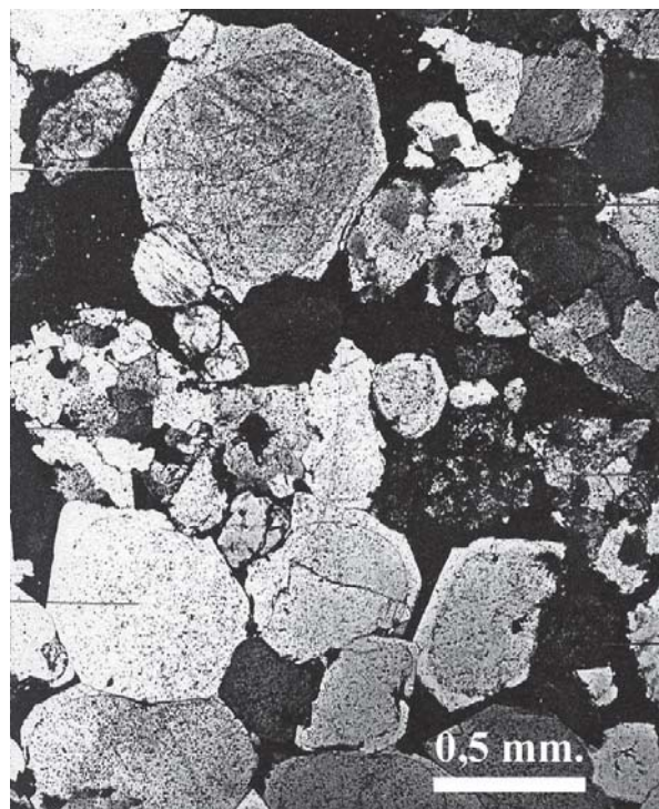
Fig. 1.- Cuarzarenita («Grès cristallisé») (Raon-l'Étape, Vosgos) (Lámina IV, Fig.14) (Cayeux, 1929).
