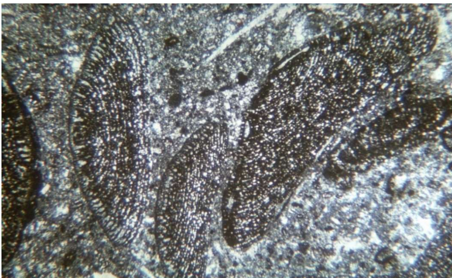
Orbitolinas
