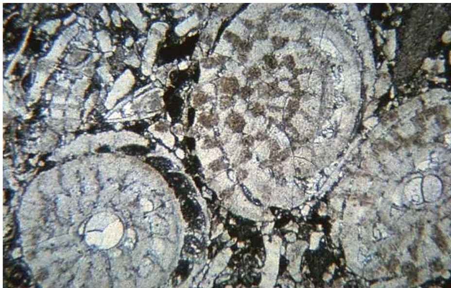
Numulites
