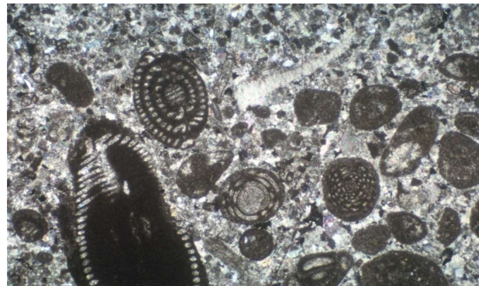
Alveolinas
