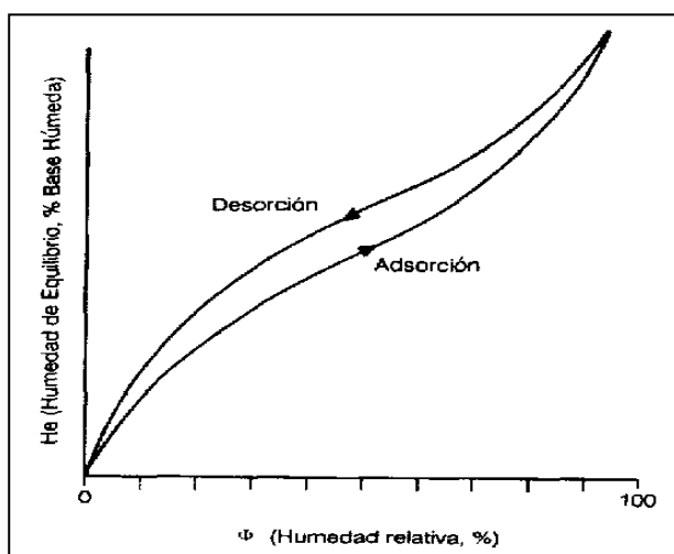
Fig. 1. Isoterma de sorción. En abscisas la humedad relativa ( H_r , %), en ordenadas el contenido en agua ( w , %). La curva superior corresponde al secado (desorción) y la inferior al mojado (adsorción). En el tramo inferior de las curvas tiene lugar el transporte de agua en fase de vapor y en el superior en fase líquida, por condensación higroscópica.
